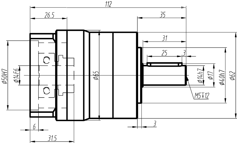
标准轴
